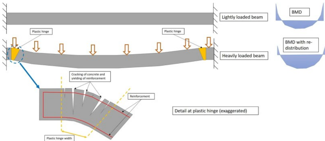
Betonové nosníky vstupující do plasticity a v místě kolapsu.
