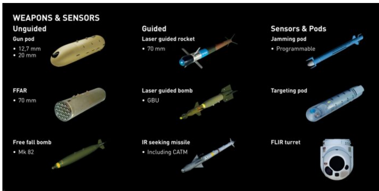
Podvěsná výzbroj českého bitevníku L-39NG
