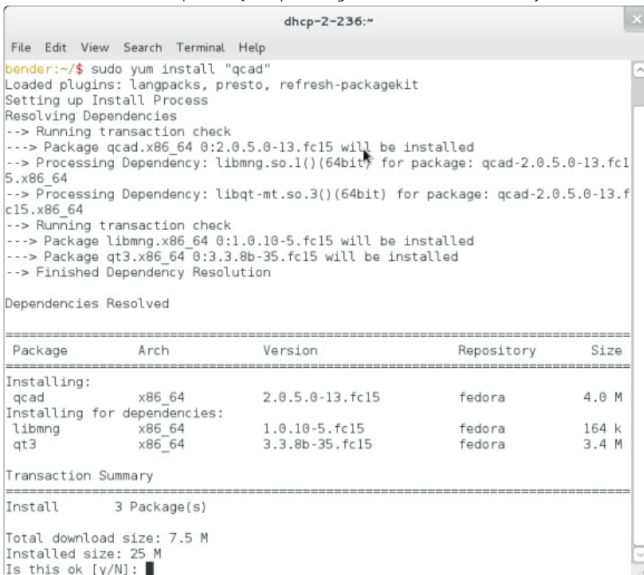
Instalace aplikace Qcad a všech knihoven, na nichž tato aplikace závisí, s využitím příkazu „yum“ spuštěného z příkazové řádky (s právy superuživatele).
