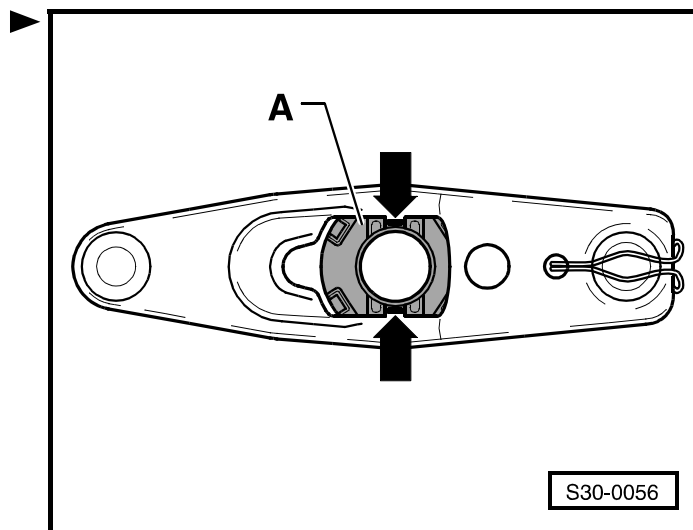
Obr. 2: Demontáž a montáž vypínacího ložiska
