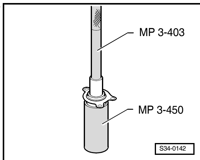
Obr. 3: Vyrazení těsnicího kroužku z vodícího pouzdra
