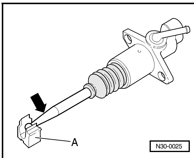
Obr. 2: Montáž ovládací tyče a hlavního spojkového válce do uchycení - A- ve - směru šipky- ►
