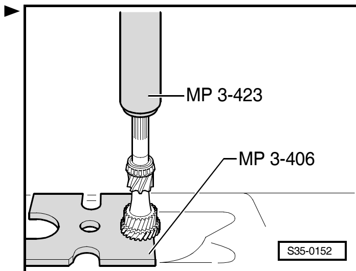
Obr. 7: Nalisování ozubeného kola 3. rychlosti
