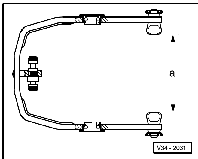
Obr. 6: Řadicí vidlička s namontovanými segmenty
