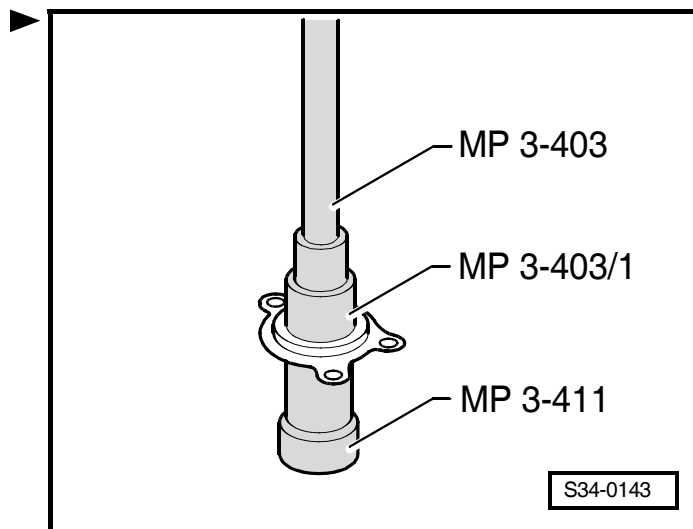
Obr. 4: Naražení těsnicího kroužku do vodícího pouzdra až nadoraz
