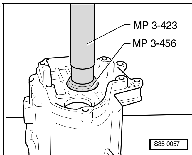
Obr. 11: Vylisování vnějšího kroužku kuželíkového ložiska ►
