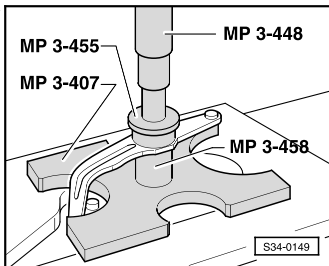
Obr. 5: Nalisování kuličkového ložiska až nadoraz
