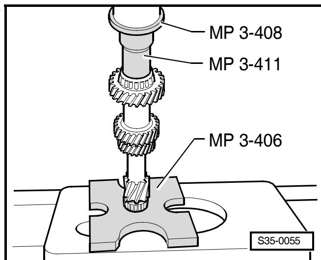
Obr. 9: Nalisování vnitřního kroužku kuželíkového ložiska ►
