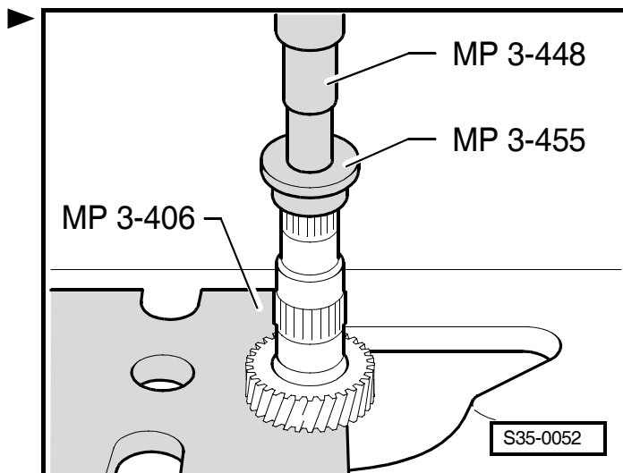
Obr. 6: Vylisování ozubeného kola 3. rychlosti
