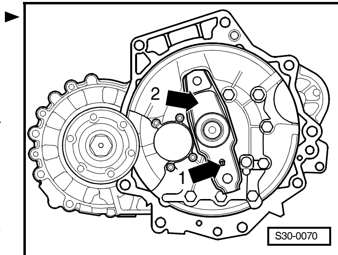
Obr. 1: Demontáž a montáž vypínací páky s vypínacím ložiskem spojky a vodícím pouzdem
